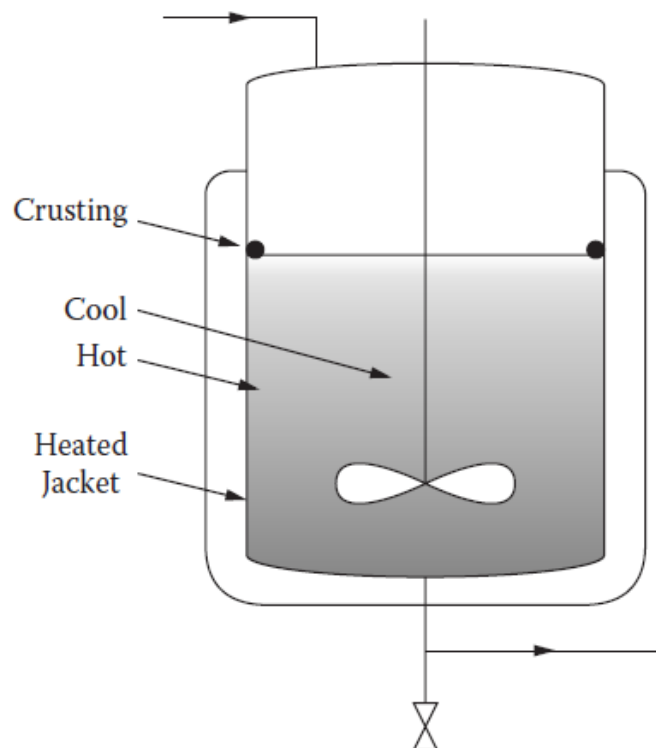
efekti zagrijavanja u scale-up reaktoru grijanom konvencionalnim načinom
